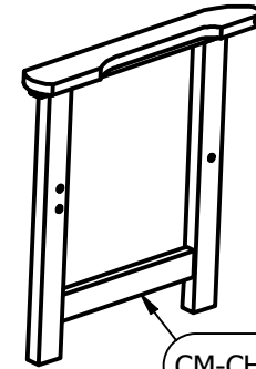
CM-CHGSQ01-ASM-004 RIGHT ARM ASSEMBLY
