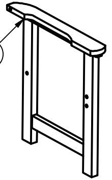
CM-CHGSQ01-ASM-005 LEFT ARM ASSEMBLY
