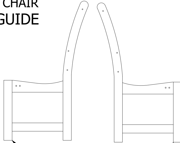
CHDL2-ASM-013 LEFT SIDE ASSEMBLY
