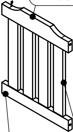
CHDL2-029 BACK TOP
